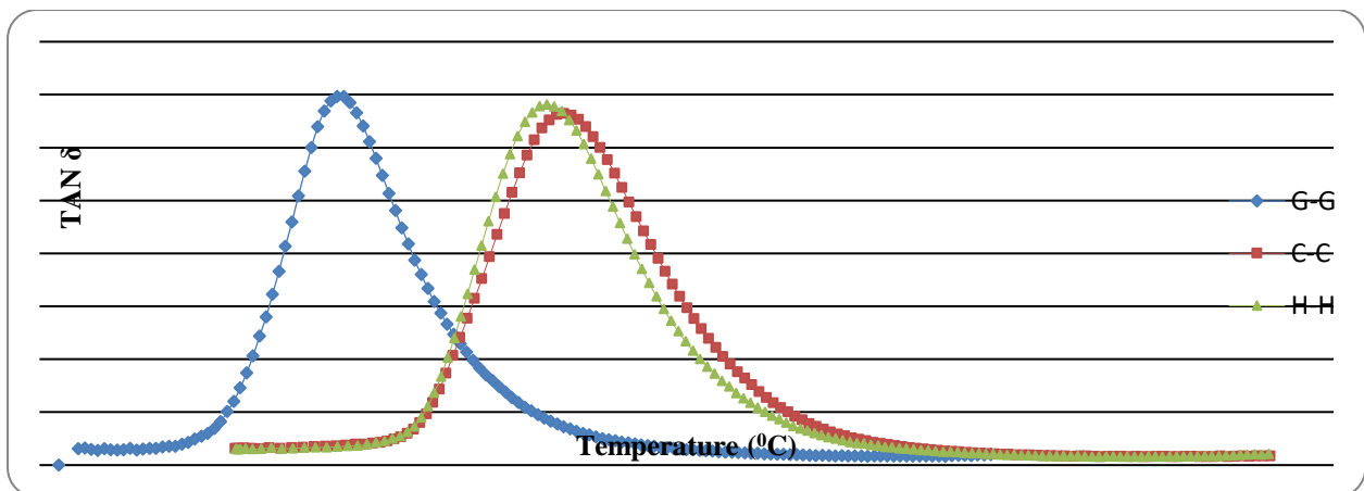
Fig: 18. Hz Tan Delta Vs Temperature
